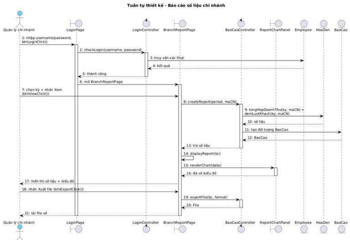
Hình. Biểu đồ tuần tự thiết kế – Báo cáo số liệu chi nhánh
