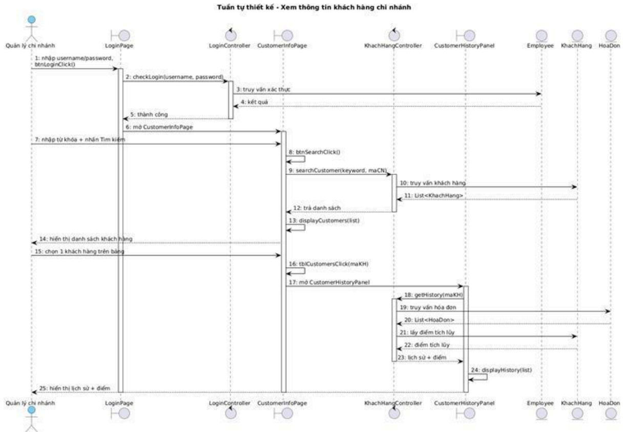
Hình. Biểu đồ tuần tự thiết kế – Xem thông tin khách hàng chi nhánh
