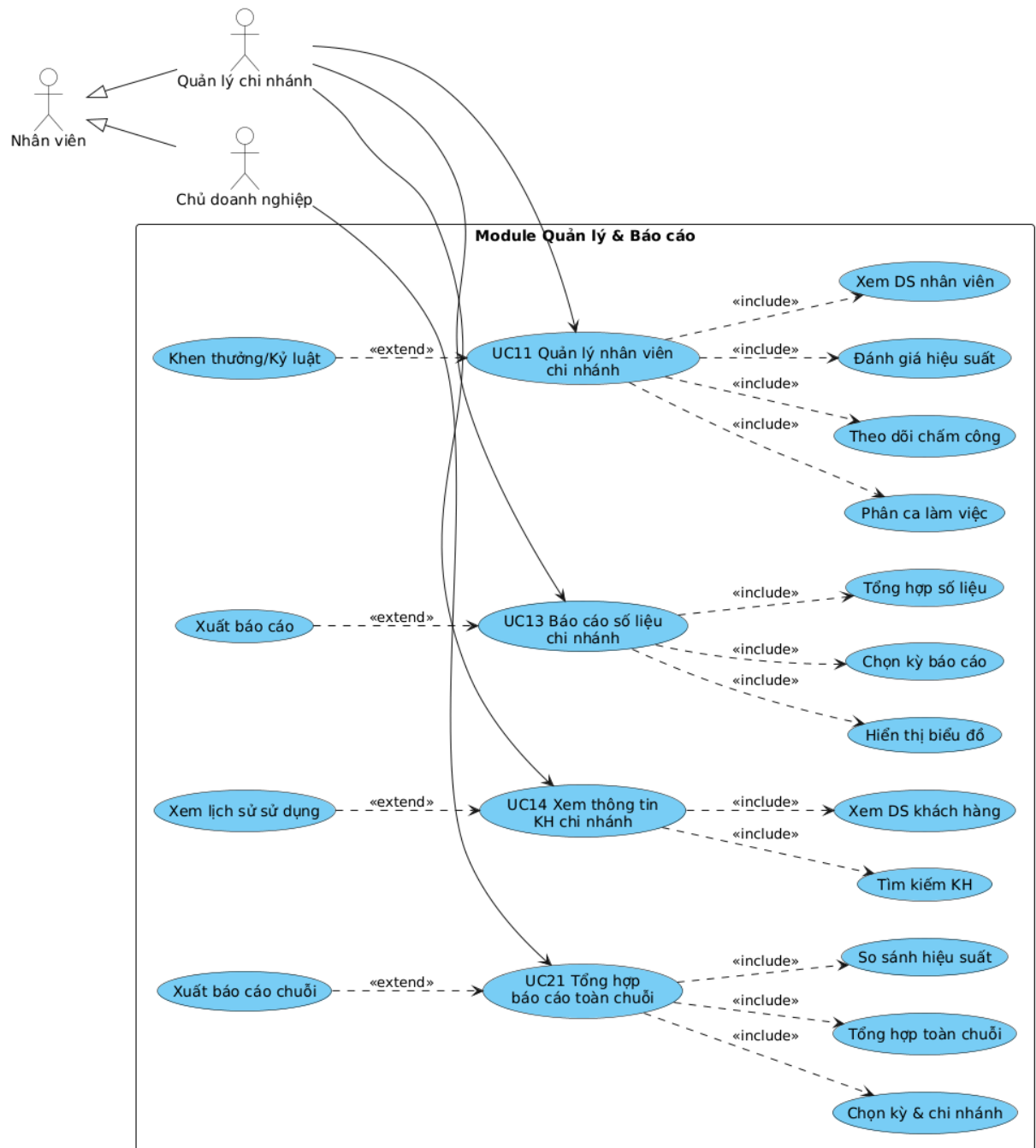
Biểu đồ Use Case chi tiết - Module Quản lý & Báo cáo (React)
